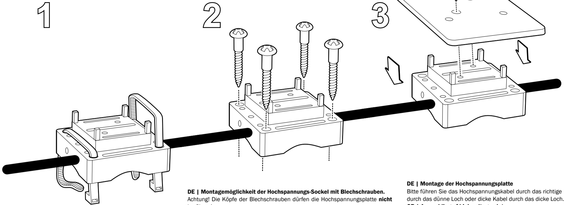
DE | Montagemöglichkeit der Hochspannungs-Sockel mit Kabelbindern. GB | Assembling option for high-voltage socket with cable straps.
